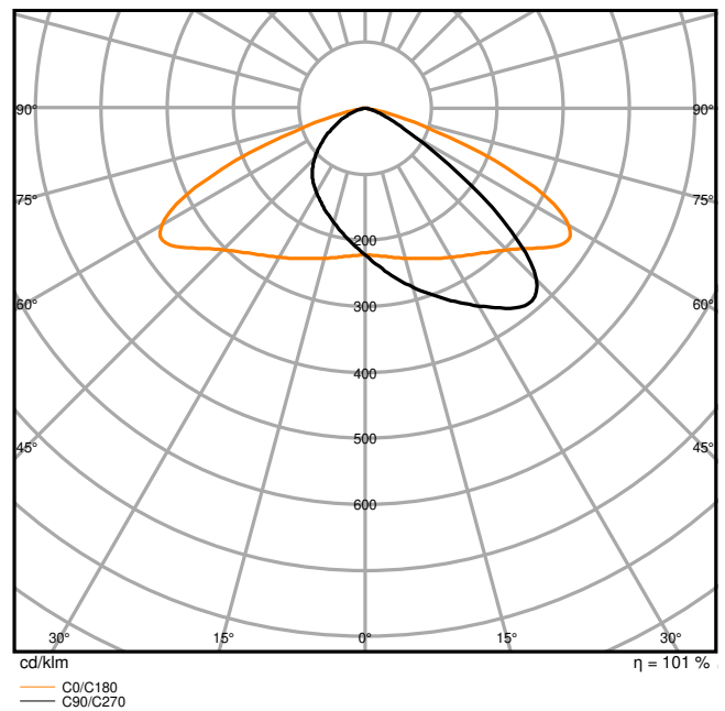
FL PFM 290W 4000K ASYM 45X140 BK
