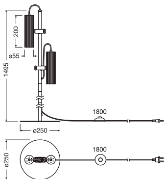
Produktmaße (in mm)
