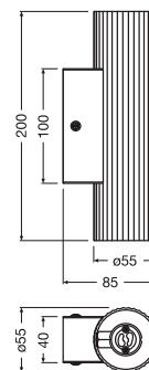
Produktmaße (in mm)
