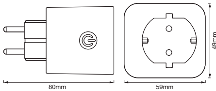
Produktmaße (in mm)
