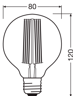
Produktmaße (in mm)
