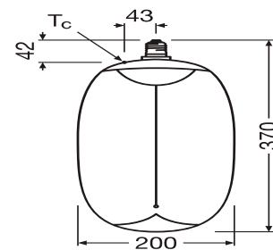
Produktmaße (in mm)
