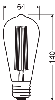
Produktmaße (in mm)
