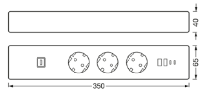
Produktmaße (in mm)
