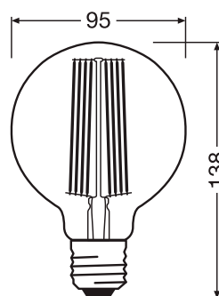
Produktmaße (in mm)
