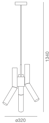
Produktmaße (in mm)
