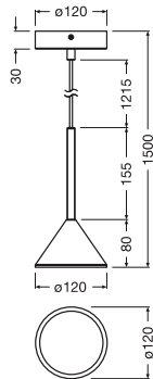
Produktmaße (in mm)
