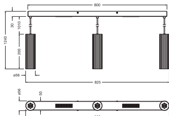
Produktmaße (in mm)
