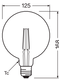
Produktmaße (in mm)
